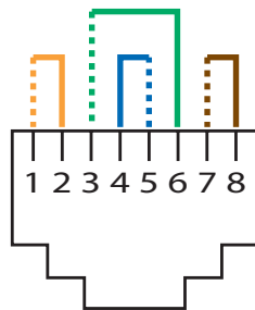
T 568 B
