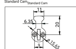
Cams
